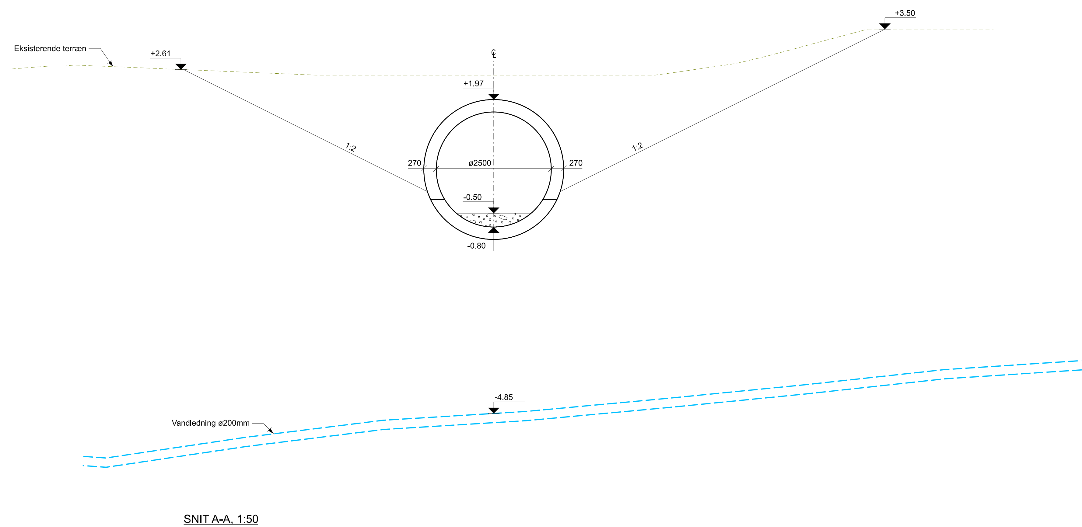
SNIT A-A, 1:50
